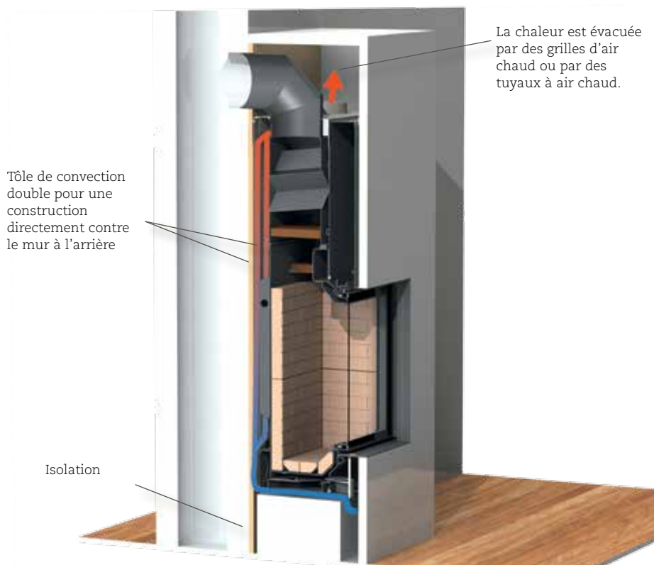
Foyer Style 62/76 k avec manteau de convection
